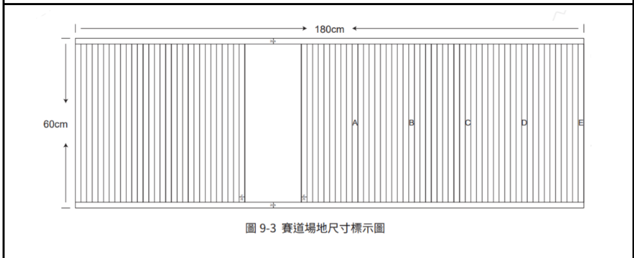
圖 9-3 賽道場地尺寸標示
